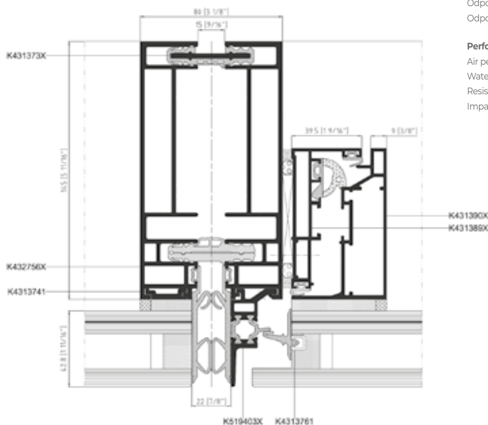
Przekrój przez słup i okno odchylne Mullion and outside opening window – cross section
